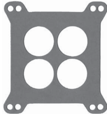
Flange Gasket - Universal H20-284 (1/16" thk.) (1 3/4" Bore)
